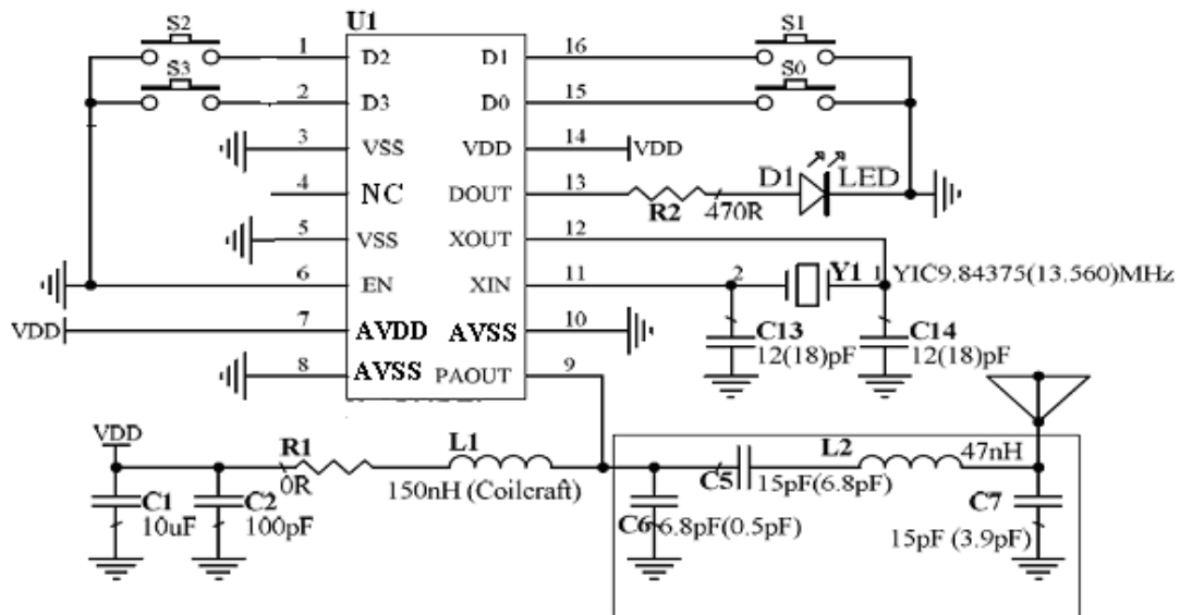
HT6P20D2T3_315(433)MHz TX
