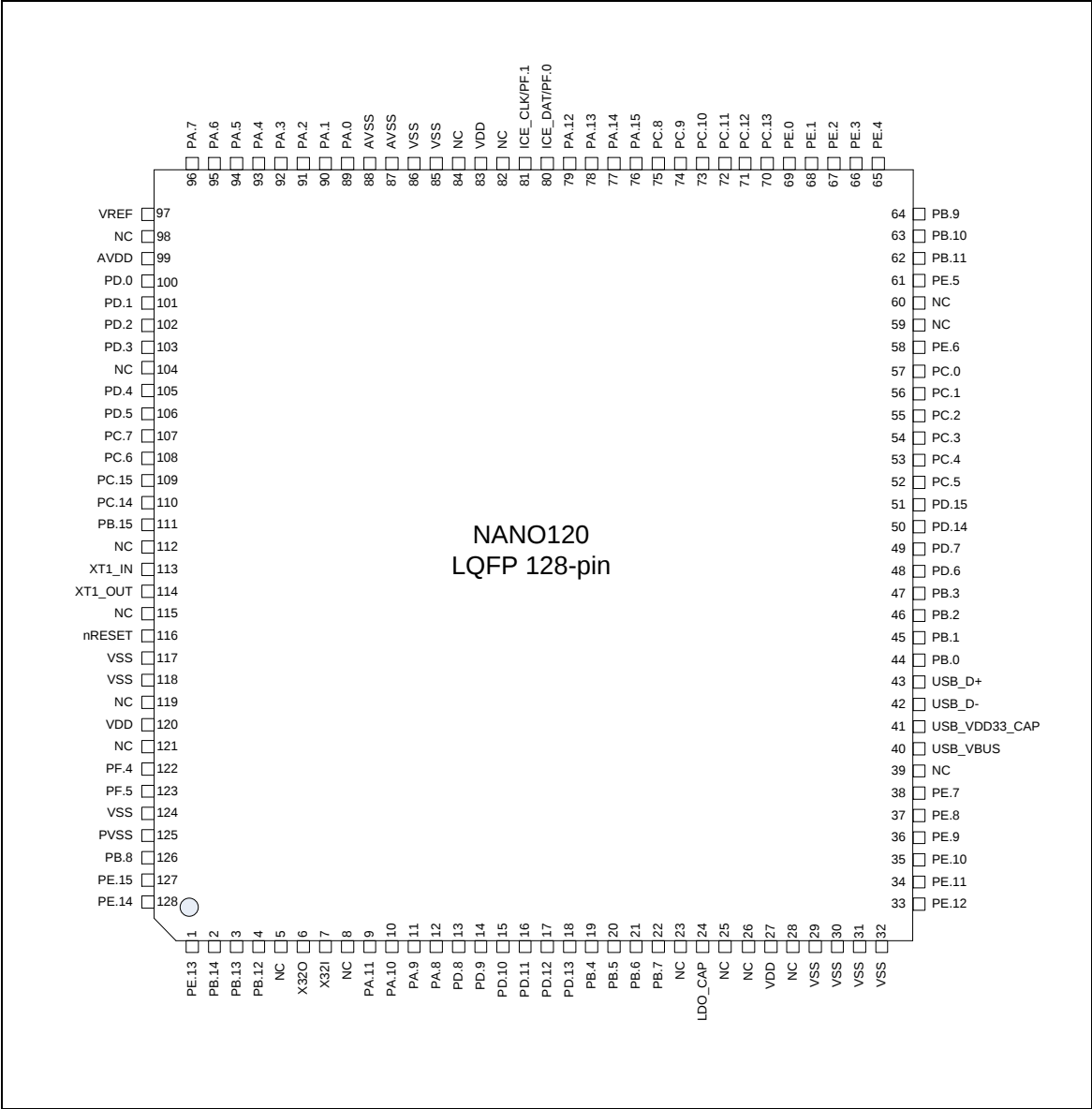
图 3-7 NuMicro® Nano120 LQFP 128-pin 管脚图
