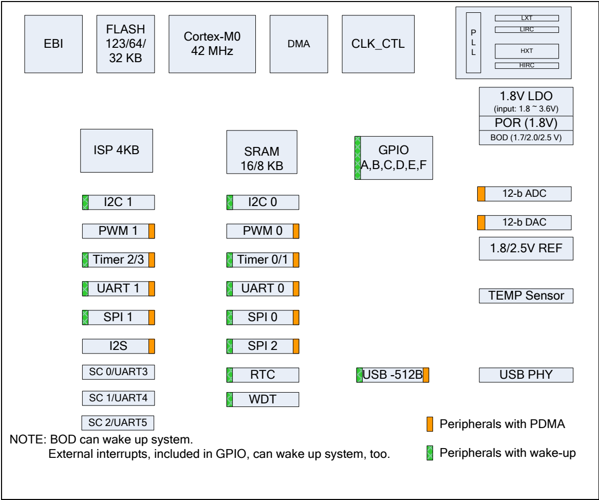
图 4-3 NuMicro® Nano120 框图
