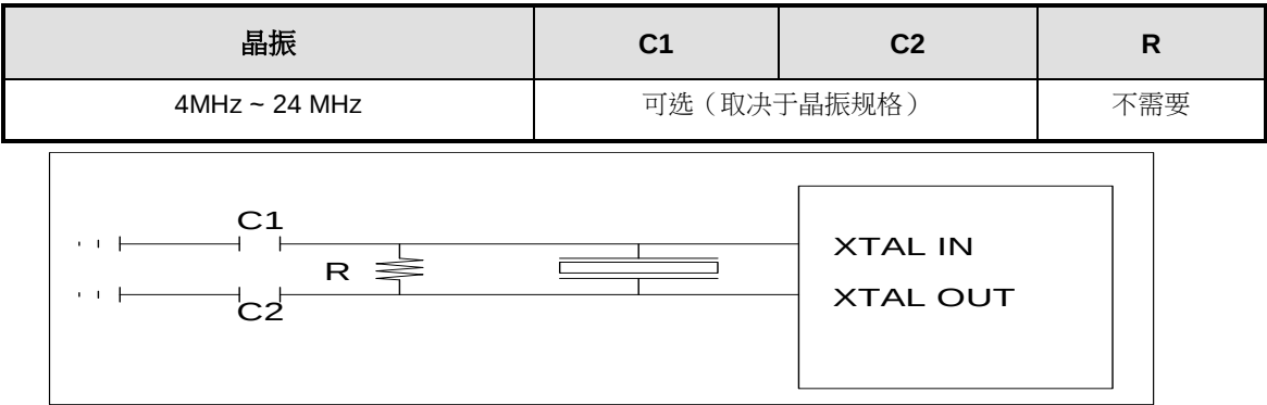
图 9-1典型晶振应用电路
