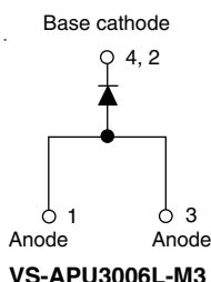
VS-APU3006L-M3
