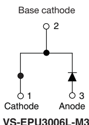
VS-EPU3006L-M3
