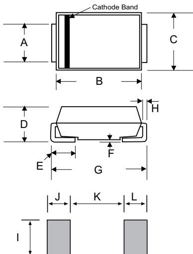
DO-214AB (SMC -Bend)
