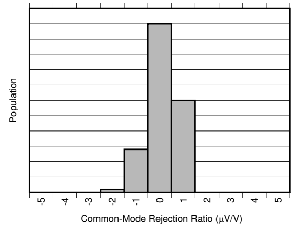
图 6-6. CMRR Distribution (INA30xA2-Q1)
