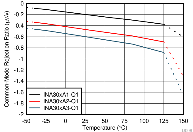
图 6-8. CMRR vs. Temperature
