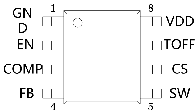
ESOP8
