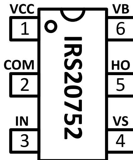
6-Lead SOT 23
