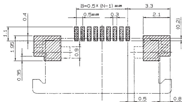
推奨基板取寸法 (コネクタ搭載側) MOUNTING LAYOUT (CONN. MOUNTING SIDE)
