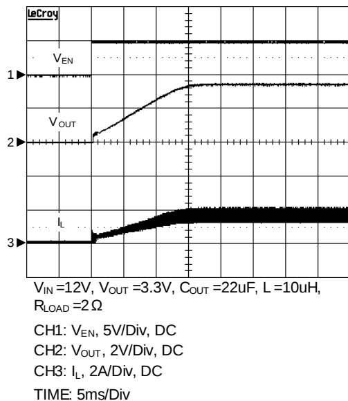
Enable
