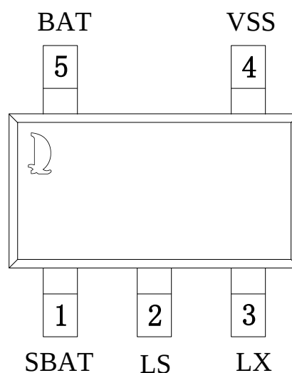
SOT23-5
