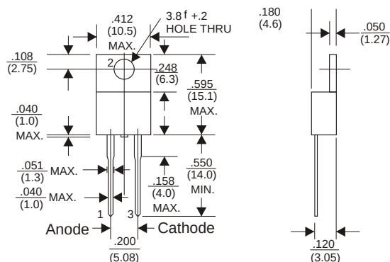
TO-220A
