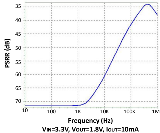
PSRR
