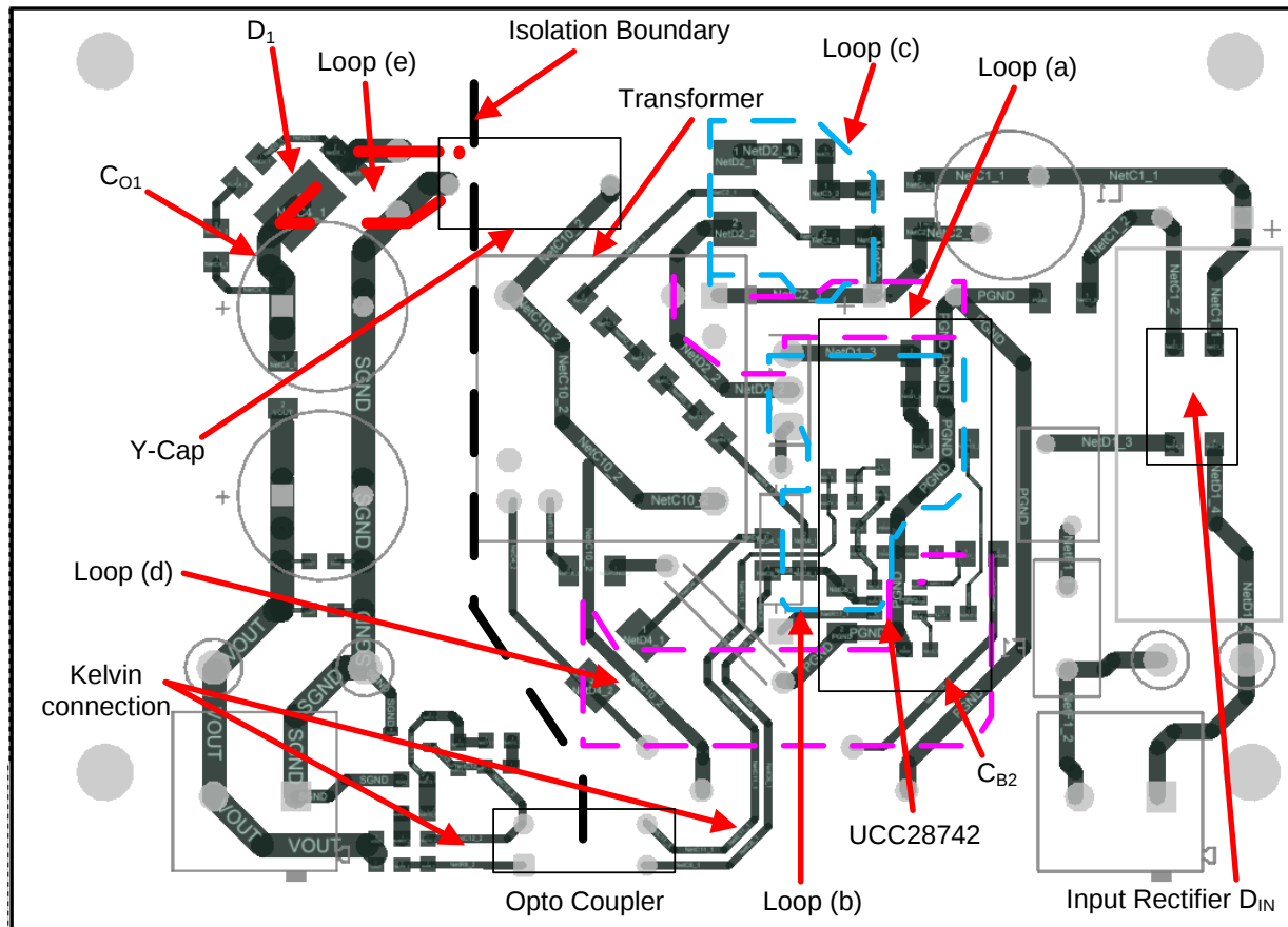
图 26. Layout Example
