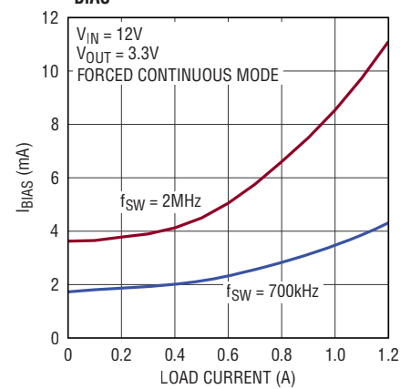
I_{BIAS} vs Load
