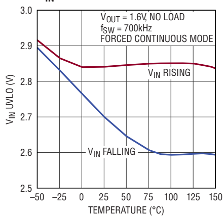
V_{IN} UVLO
