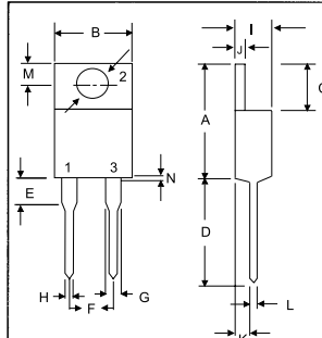
TO-220A
