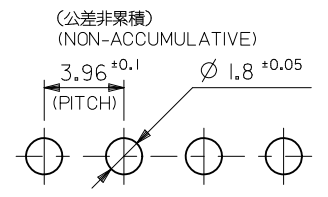
基板取付穴推奨寸法 RECOMMENDED P.C.BOARD HOLE DIM.
