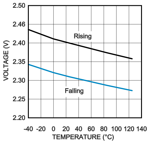
POR Threshold
