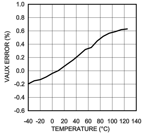
VAUX Error, VAUX=1V
