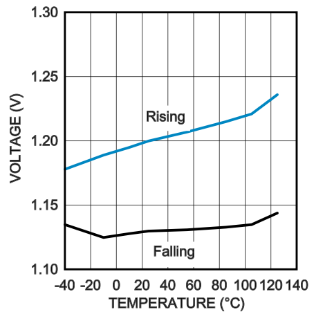
ENABLE Threshold
