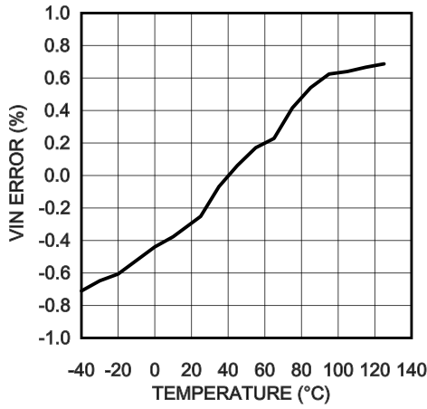
VIN Error, VIN=12V
