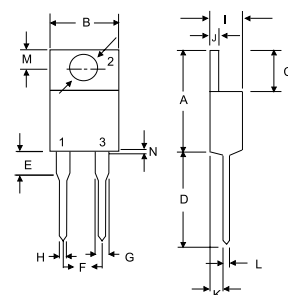
TO-220A
