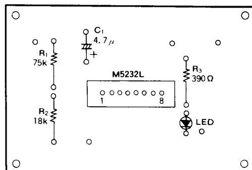
(PARTS SIDE)
