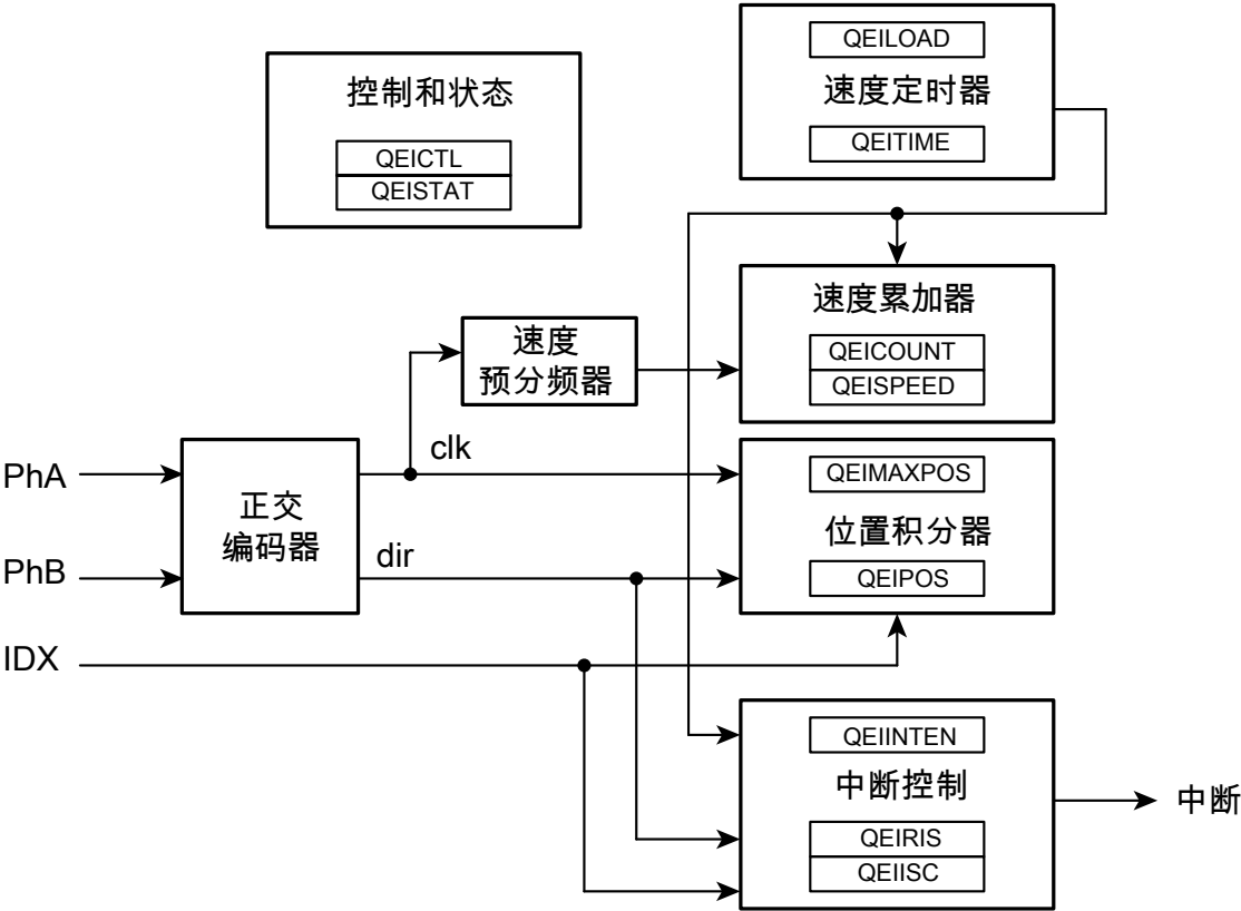
图 19-1. QEI结构图
