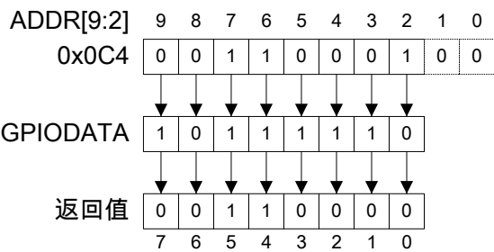
图 9-4. GPIODATA 读实例
