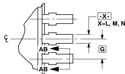
VIEW Y
