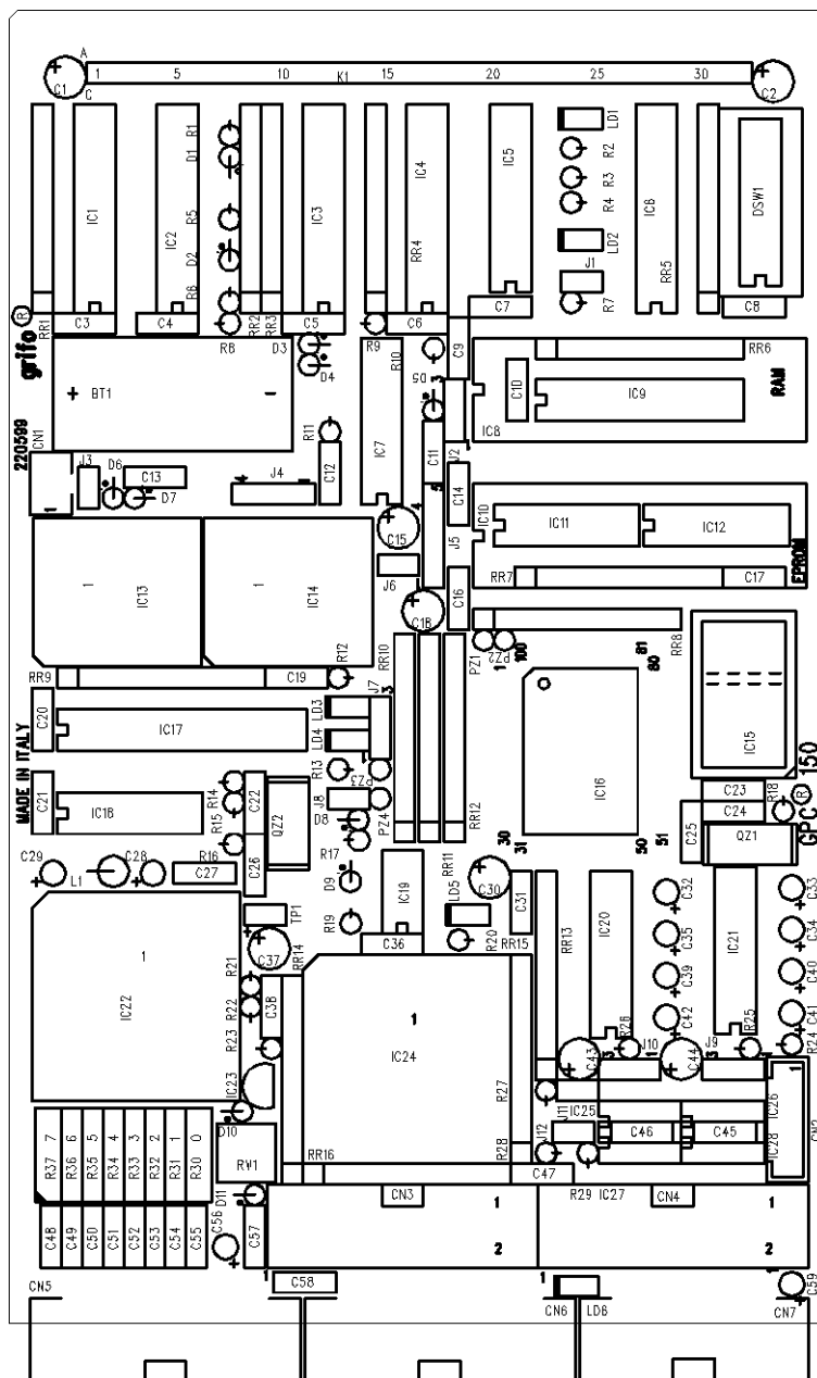
FIGURA 33: PIANTA COMPONENTI
