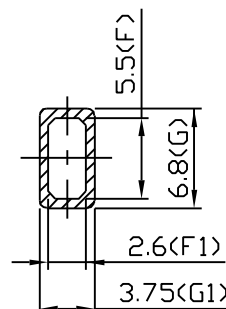
SEC A-A
