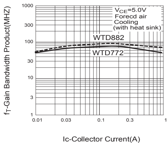
F9. f_T - I_C
