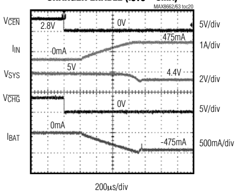
CHARGER ENABLE ( I_{SYS} = 0mA )
