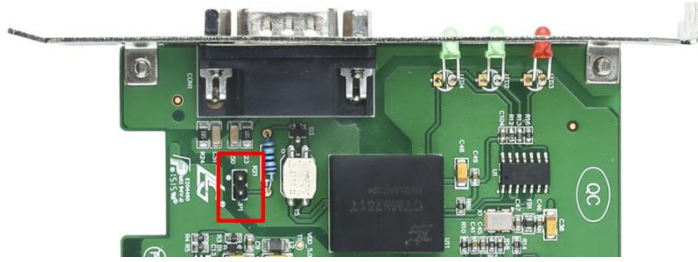
图 2.2 终端电阻选择示意图
