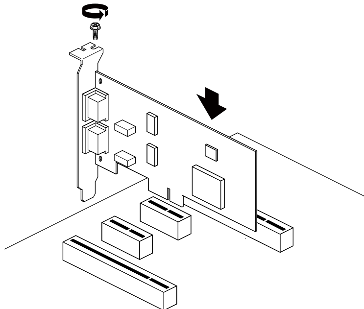
图 2.3 PCIe-9110I 系列 CAN 接口卡
