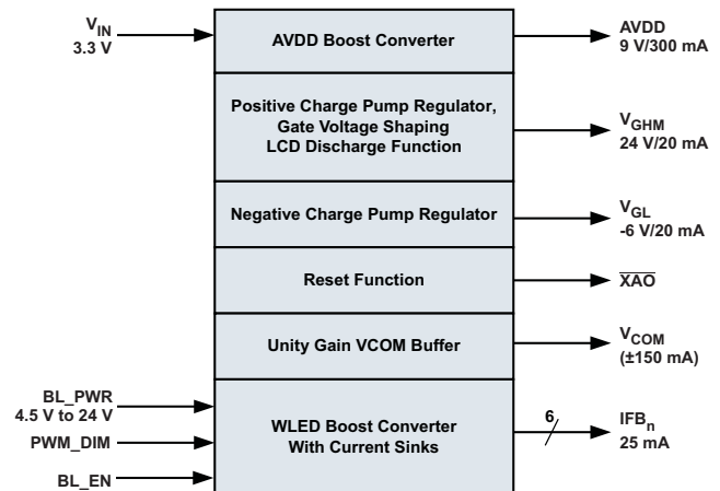
简化框图
