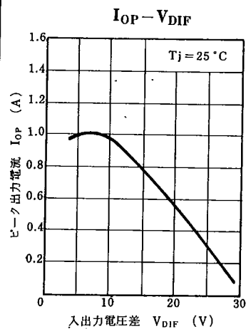
共通特性図
