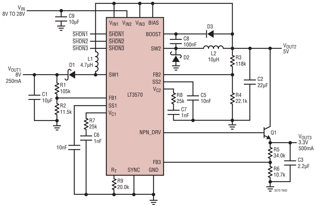
DSL Modem
