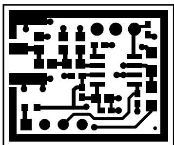
Figure 7a. Top Layer
