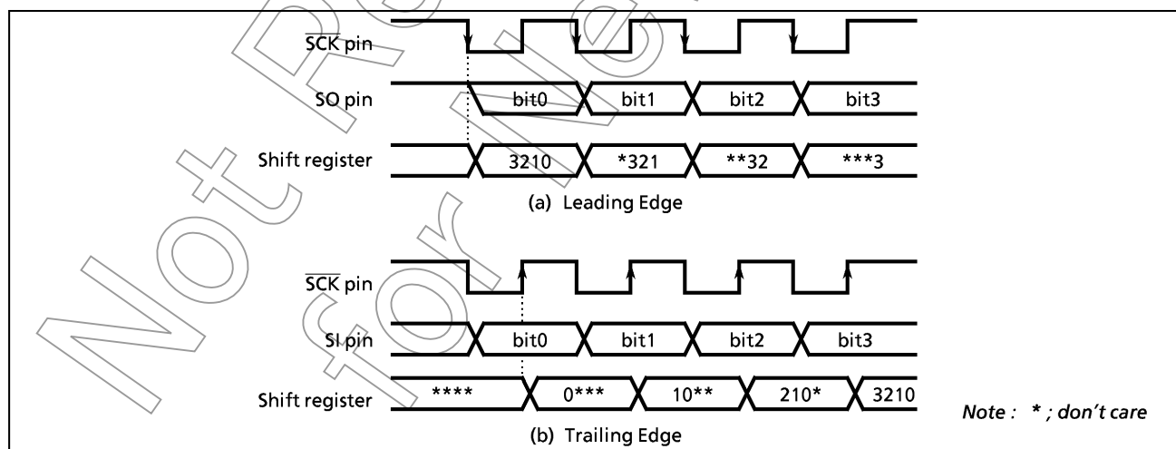
Figure 2-39. Shift Edge
