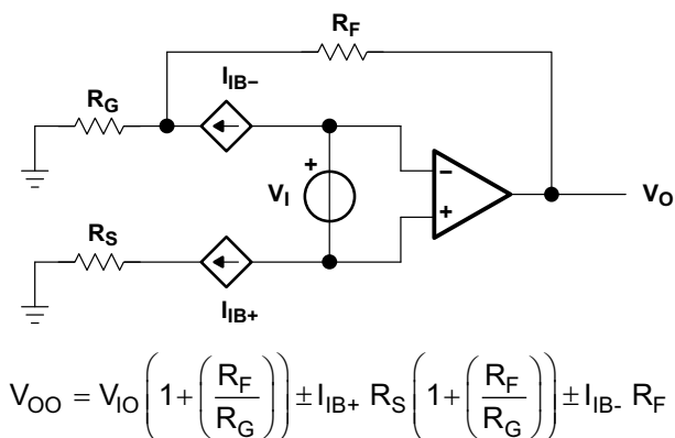
图 29. 输出失调电压模型
