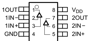
引脚功能: TLV2372-Q1
