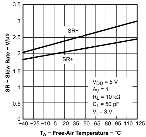
图 18. 压摆率与自然通风温度间的关系
