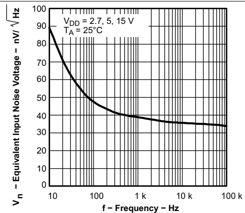
图 20. 等效输入噪声电压与频率间的关系
