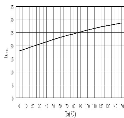
h_{FE} - T_a
