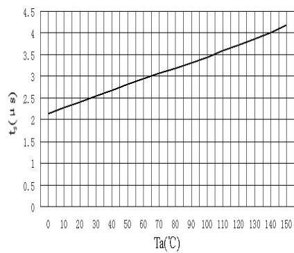
t_S - T_a
