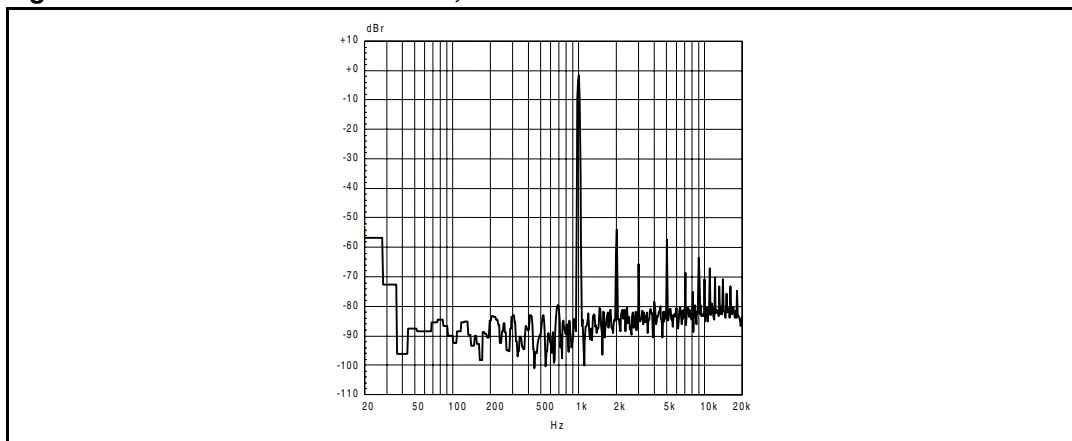
Figure 42. FFT -60 dB SE 1 kHz SE, 2 \Omega
