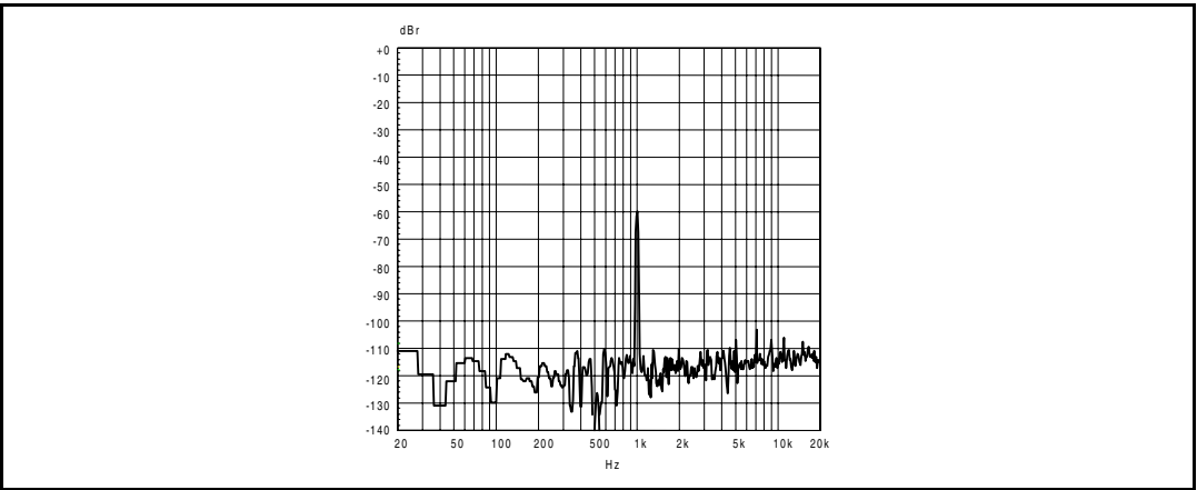
Figure 44. FFT -60 dB SE 1 kHz SE, 3 Ω
