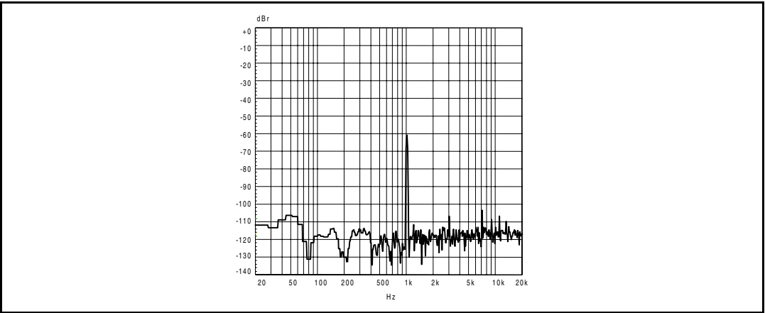
Figure 43. FFT -60 dB SE 1 kHz SE, 4 Ω
