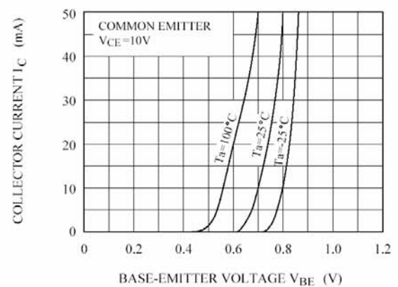
I_C - V_{BE}
