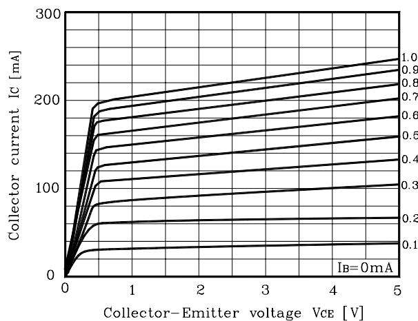
Fig. 4 I_C - V_{CE}
