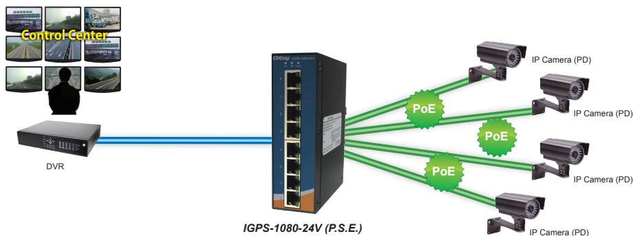
IGPS-1080-24V (P.S.E.)
