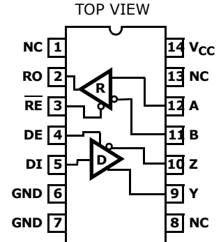
ISL3150E, ISL3153E, ISL3156E (14 LD SOIC)
