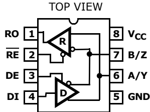
ISL3152E, ISL3155E, ISL3158E (8 LD MSOP, 8 LD SOIC, 8 LD PDIP)
