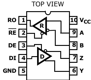
ISL3150E, ISL3153E, ISL3156E (10 LD MSOP)
