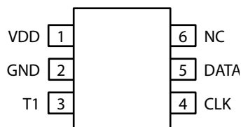
SOT23-6
