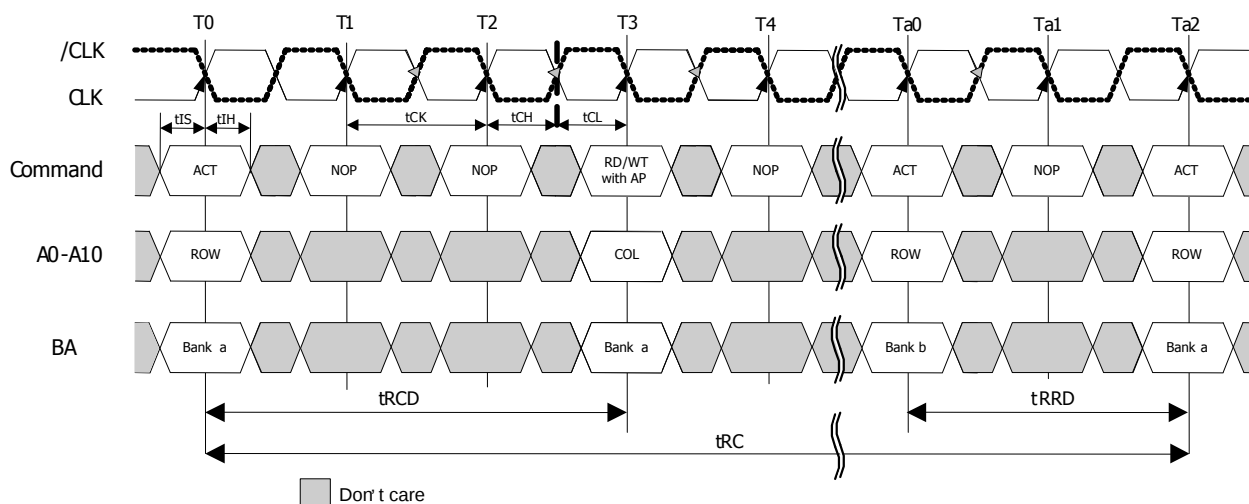
Figure11 : t RC , t RRD , t RC
