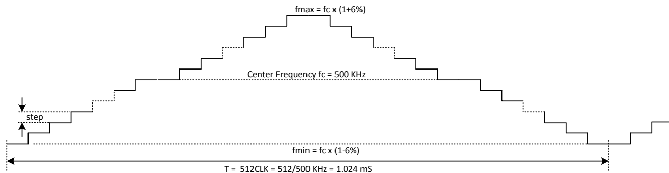
图 7-3. 展频频谱图
