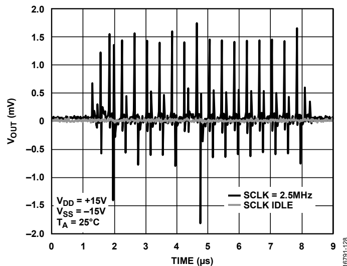
图28. 数字馈通
