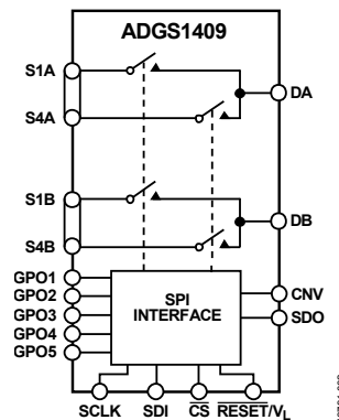
图2. ADGS1409功能框图
