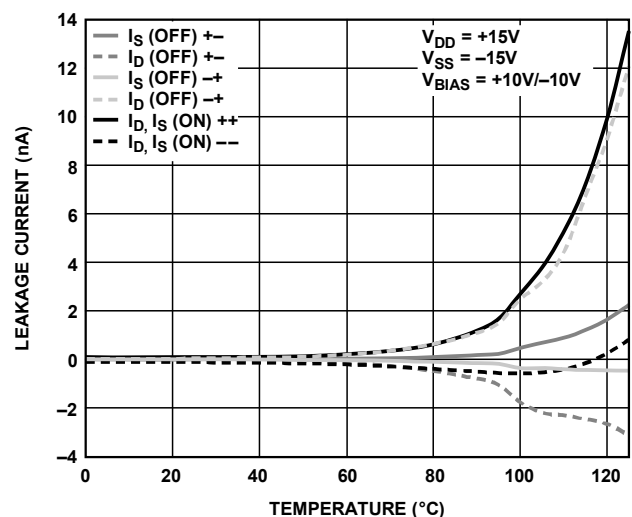
图16. 漏电流与温度的关系 (±15 V双电源)
