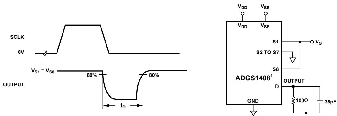
图39. 先开后合时间延迟, t_D
