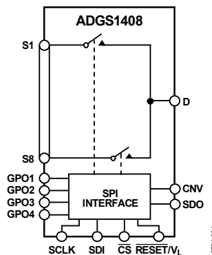
图1. ADGS1408功能框图
