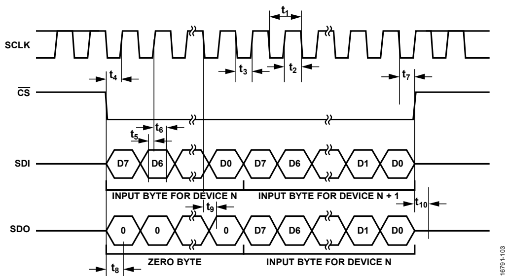
图4. 菊花链时序图
