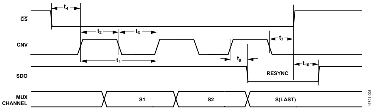
图6. 轮询时序图
