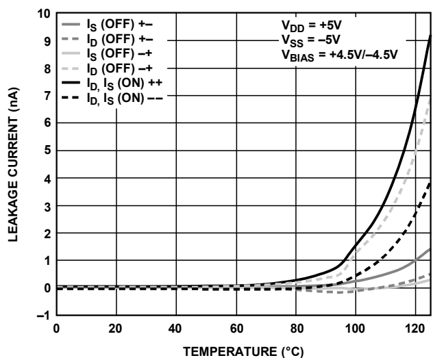
图17. 漏电流与温度的关系 (±5 V双电源)
