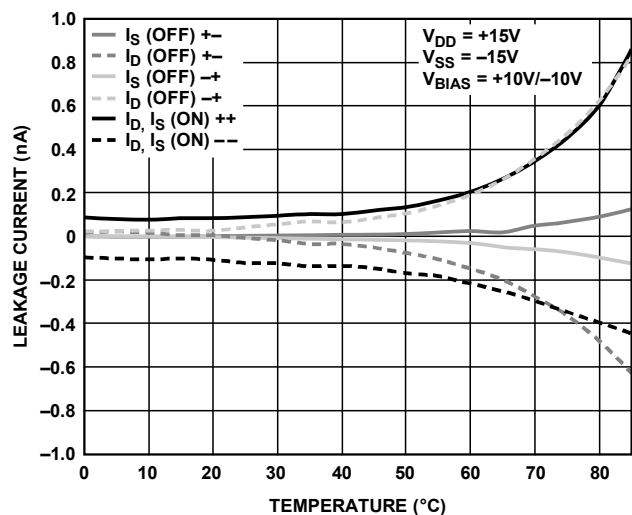
图15. 漏电流与温度的关系 (±15 V双电源)
