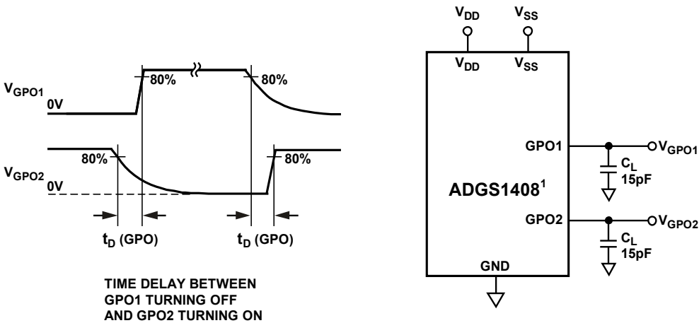
图44. GPOx先开后合时间延迟, t_D(GPO)
