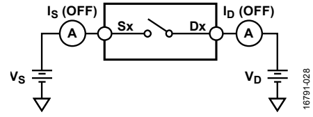
图35. 关断泄漏
