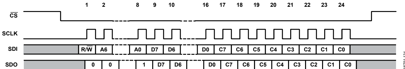
图46. CRC使能后的时序图
