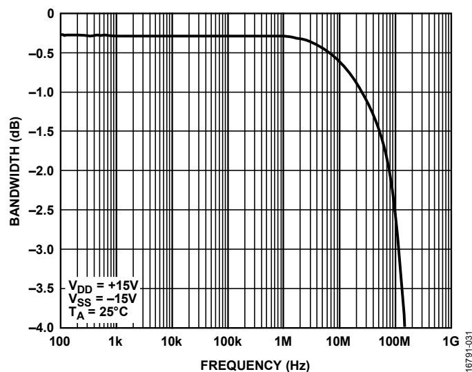
图27. ADGS1409插入损耗与频率的关系 ( \pm 15V 双电源)
