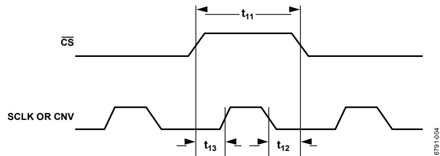
图5. SCLK或CNV和CS时序关系
