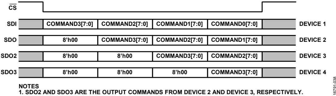
图50. 四个ADGS1408/ADGS1409器件以菊花链模式连接时的SPI帧示例
