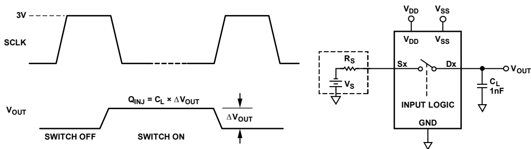
图42. 电荷注入, Q_{\text{INJ}}
