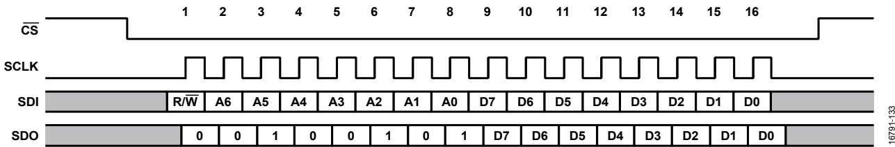
图45. 寻址模式时序图
