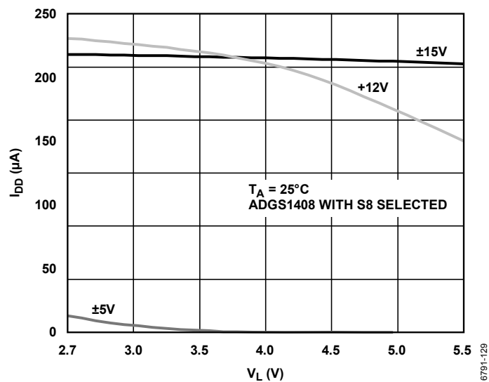
图29. I_{DD} 与 V_L 的关系
