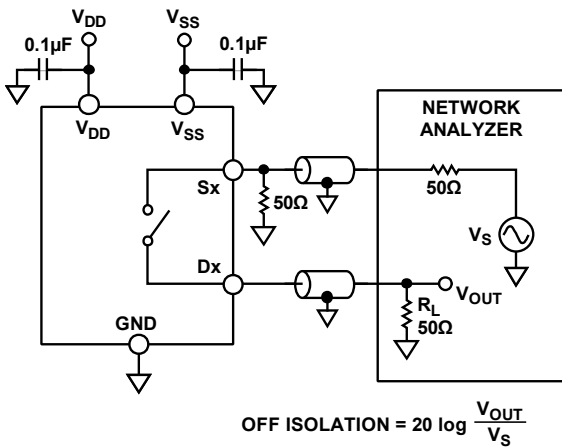
图34. 关断隔离
