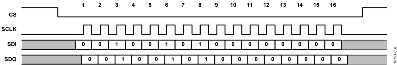
图49. 用于进入菊花链模式的SPI命令
