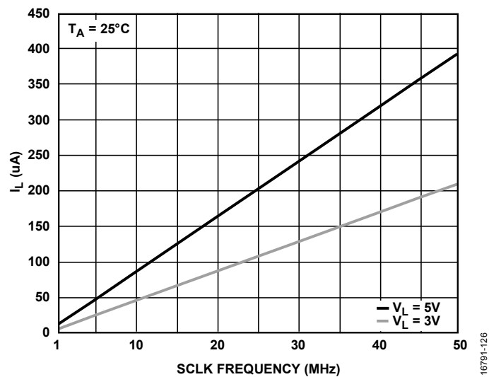
图30. I_L 与 SCLK 频率的关系 ( \overline{CS} 为高电平时)
