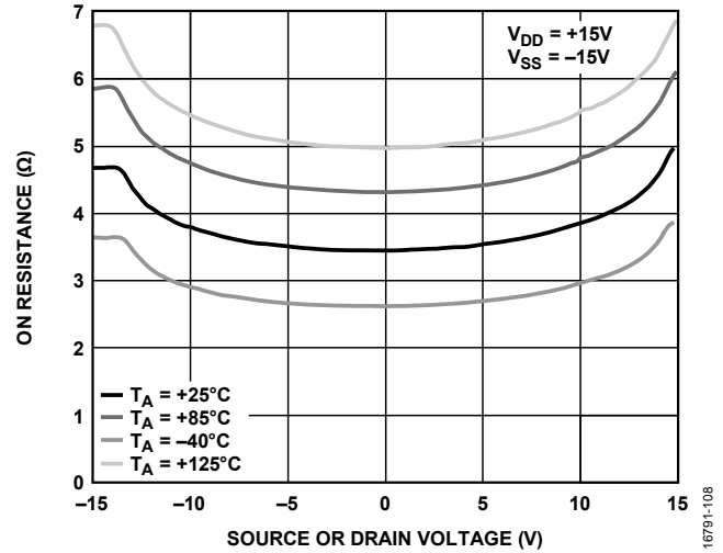
图12. 不同温度下导通电阻与 V_S 或 V_D 的关系 ( \pm 15\text{V} 双电源)
