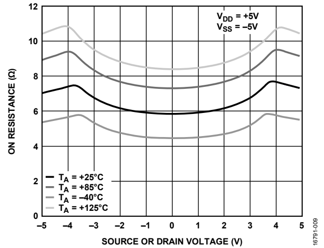
图13. 不同温度下导通电阻与 V_S 或 V_D 的关系 ( \pm 5\text{V} 双电源)
