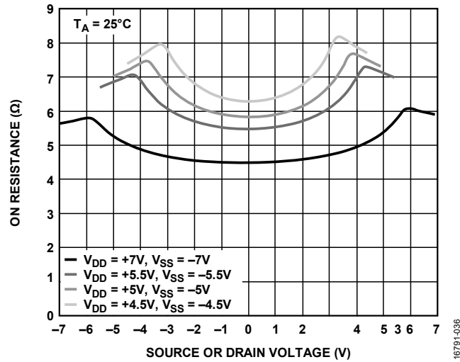
图10. 不同双电源下导通电阻与 V_S 或 V_D 的关系
