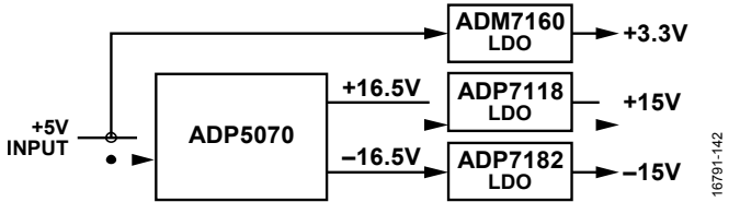
图54. 双极性电源解决方案
