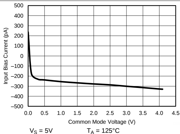
图 12. 输入偏置电流与共模电压间的关系
