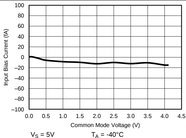
图 8. 输入偏置电流与共模电压间的关系
