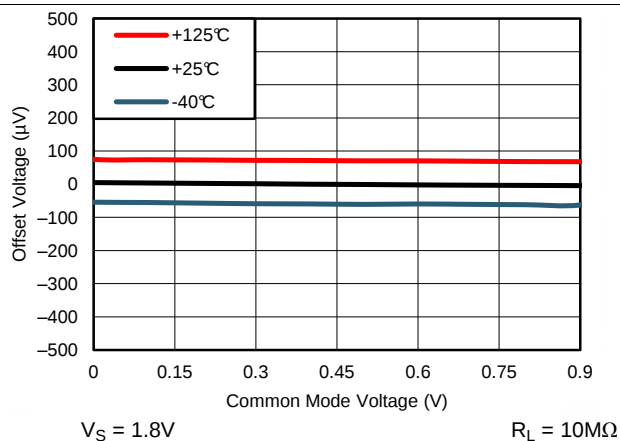
图 3. 典型偏移电压与共模电压间的关系
