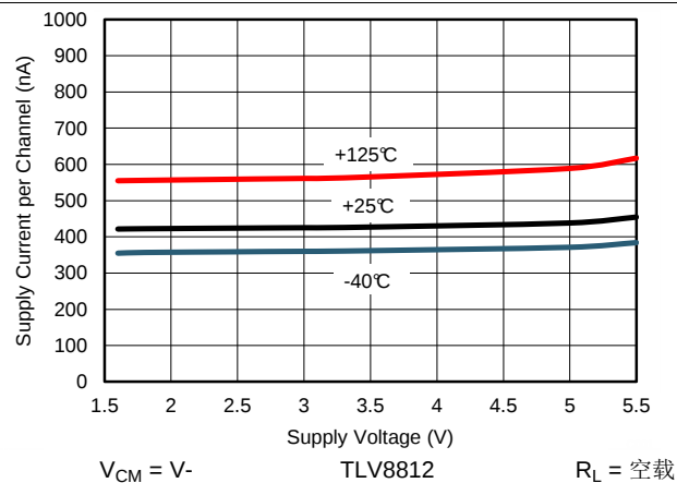
图 2. 电源电流与电源电压间的关系, TLV8812
