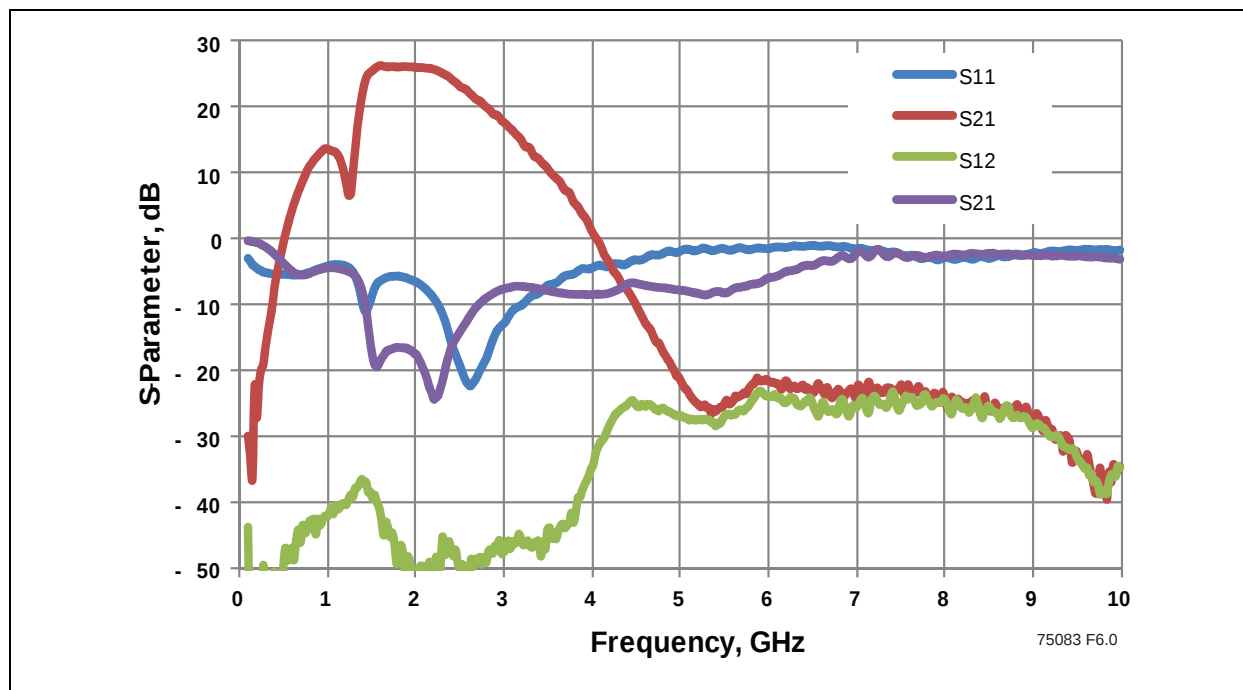
FIGURE 6-1: S-PARAMETERS
