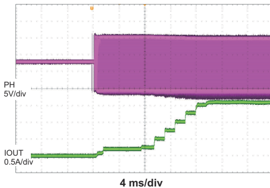
图 8-3. Current Soft Start
