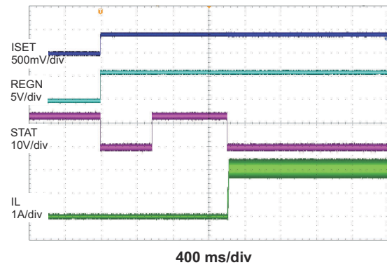
图 8-2. Charge Enable by ISET
