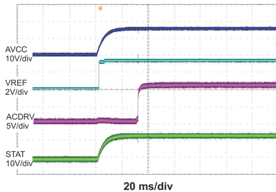
图 8-1. Power Up (ISET = 0)
