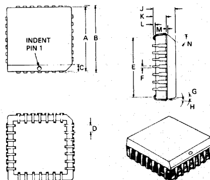
Fig. 9 FX204LH Package
