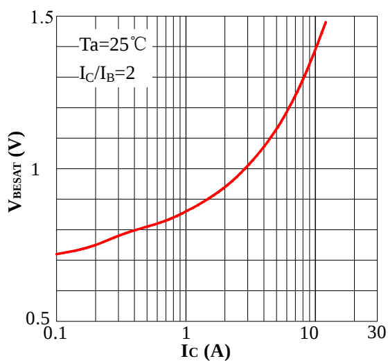
Fig6 VBESat-IC
