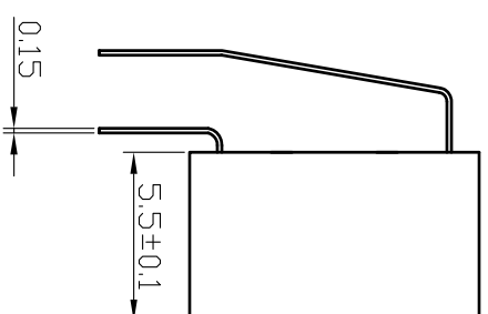
平推钮 (R)
