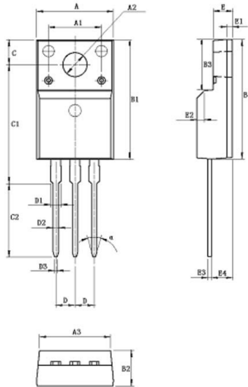
ITO-220AB
