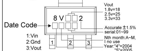
SOT-223
